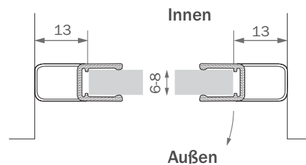
Ansicht Z
