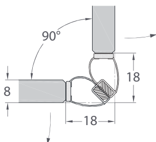
Ansicht Z
