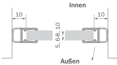
Ansicht Z
