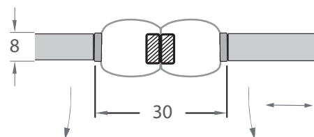
Ansicht Z
