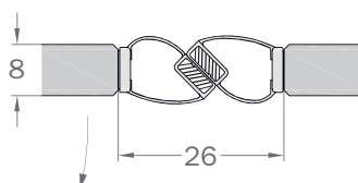
Ansicht Z
