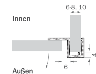
Ansicht Z
