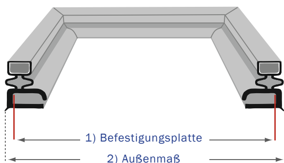
Schraubprofil
