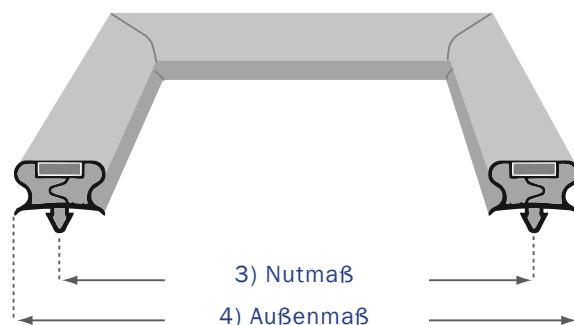
Steckprofil
